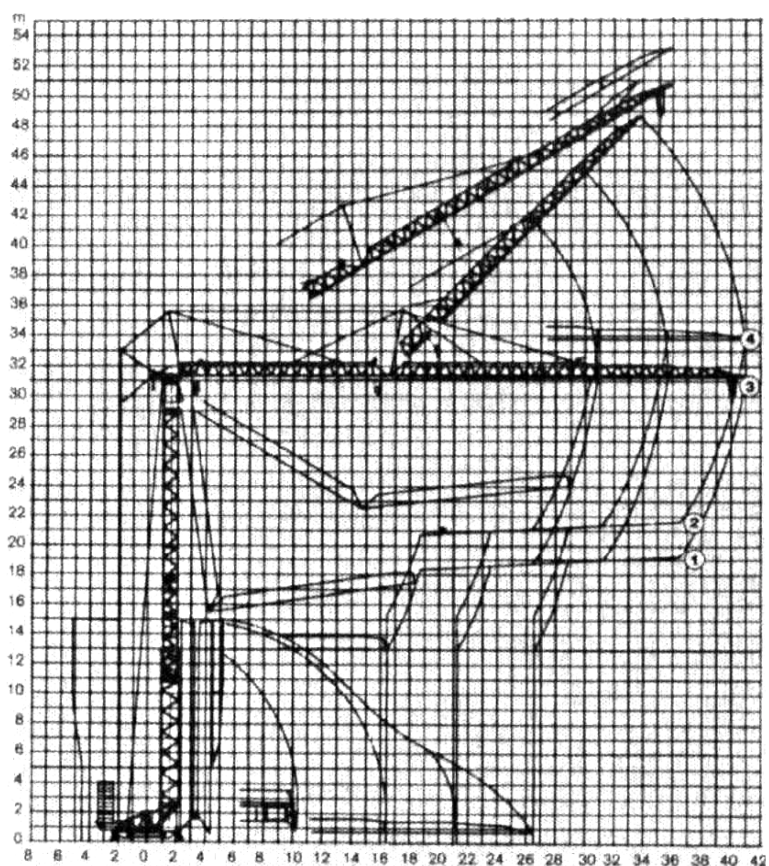
Montaż - diagram potrzebnego miejsca
